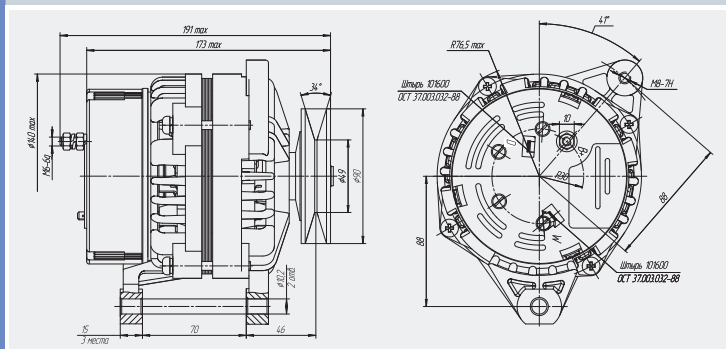
Генератор Alternator
