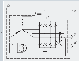
Генератор Alternator
